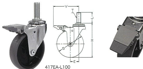
417EA-L100
